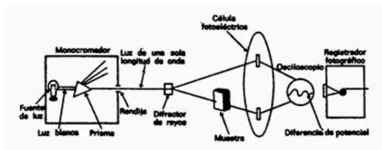
Fig. 12.2. Un espectrofotómetro. El haz de luz es dividido en dos, de tal modo que uno de los haces pase a través de la muestra que se está analizando y el otro incida directamente sobre la célula fotoeléctrica. Puesto que el haz de menor intensidad que ha atravesado la muestra libera menos electrones en la célula fotoeléctrica de lo que lo hace el haz no absorbido, los dos haces crean una diferencia de potencial que mide la cantidad de luz absorbida por la muestra.
