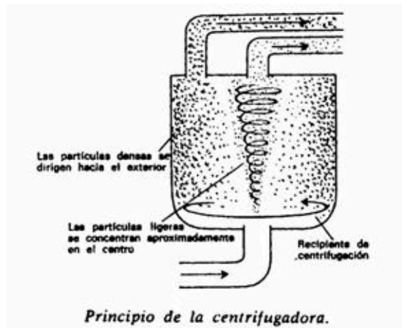
Fig. 12.1. Principio de la centrifugadora.
