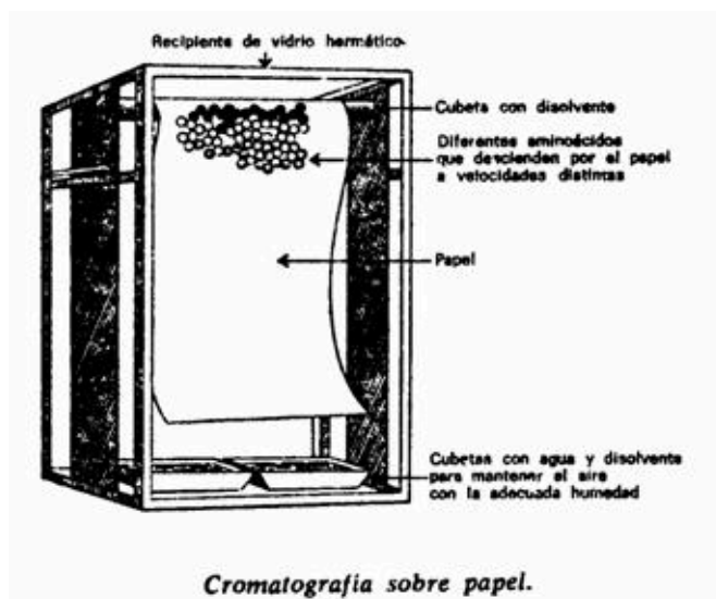
Fig. 12.3. Cromatografía sobre papel
