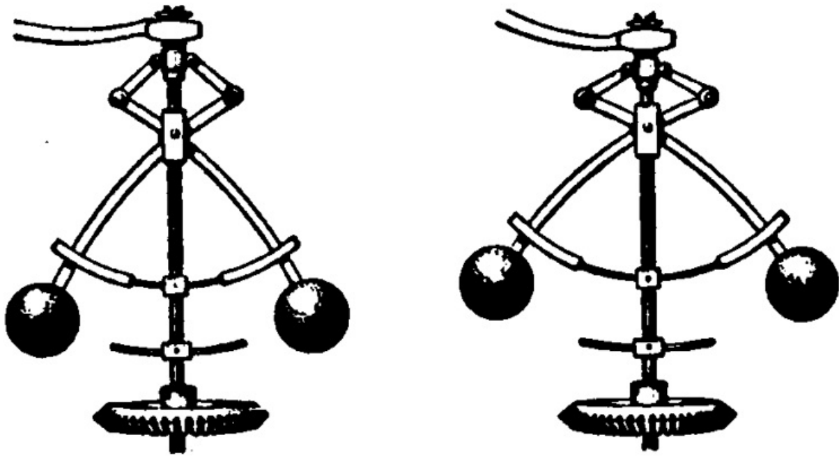
Fig. 17.4. Regulador de Watt.
