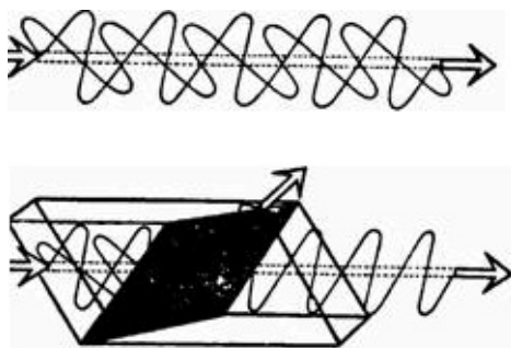
Fig. 11.1. La polarización de la luz. Las ondas de la luz vibran normalmente en todos los planos (arriba). El prisma de Nicol (abajo) permite que las vibraciones se produzcan sólo en un plano, reflejando las otras. La luz transmitida se halla polarizada en un plano.
