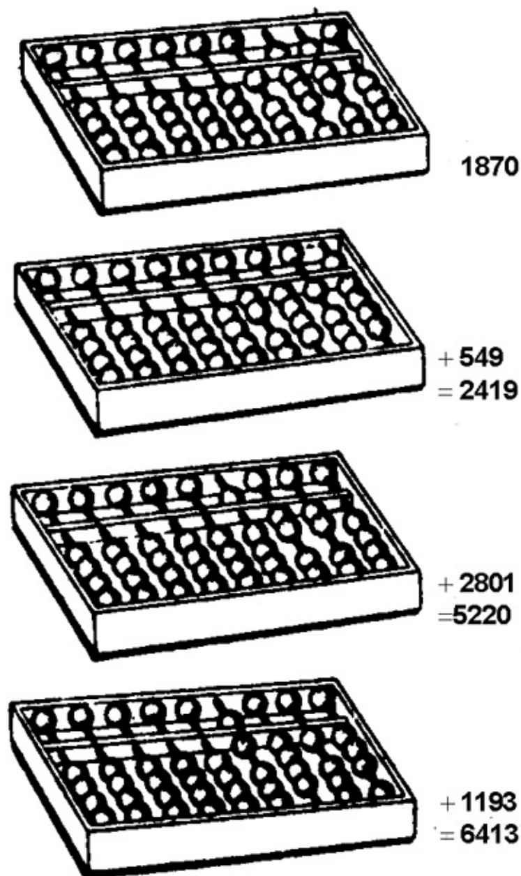
Fig. 17.5. Sumando con un ábaco. Cada bola bajo la barra vale por 1; cada bola sobre la barra vale por 5. Una bola marca una cantidad al ser movida hacia la barra. En el cuadro que aparece en la parte superior, la columna de la derecha señala 0; la que está a la izquierda de ésta señala 7 o (5 + 2); la que está a su lado marca 8 o (5 + 3); el contiguo 1: la cifra resultante es, pues, 1870. Si a esta cantidad se añade 549, la columna de la derecha se convierte en 9 o (9 + 0); la siguiente suma (4 + 7) se convierte en 1, llevándose 1; y la cuarta suma es 1 + 1, o 2; la suma arroja 2.419, según muestra el ábaco. La simple maniobra de llevarse 1 moviendo hacia arriba una bola en la columna adjunta posibilita calcular con gran rapidez; un operador experto puede sumar con más rapidez que una máquina sumadora, según quedó demostrado en una prueba efectuada en 1946.
