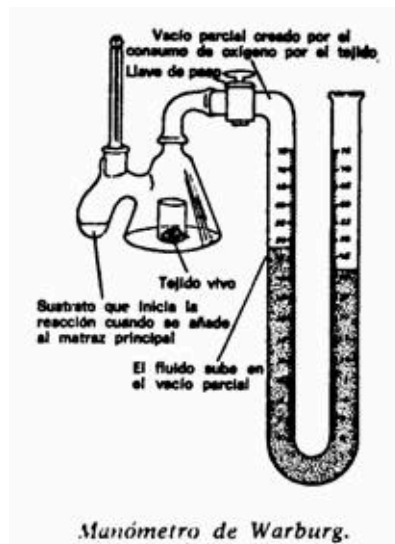
Fig. 12.4. Manómetro de Warburg.
