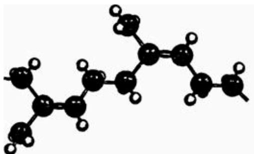
Fig. 11.3. La molécula de gutapercha, una porción de la cual se muestra aquí, está formada por miles de unidades de isopreno. Los primeros cinco átomos de carbono en la izquierda (esferas negras) y los ocho átomos de hidrógeno unidos a ellos forman una unidad de isopreno.
